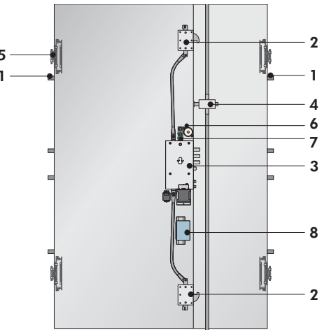
Sleek Next Elettra Doppio Battente - Double Leaf
