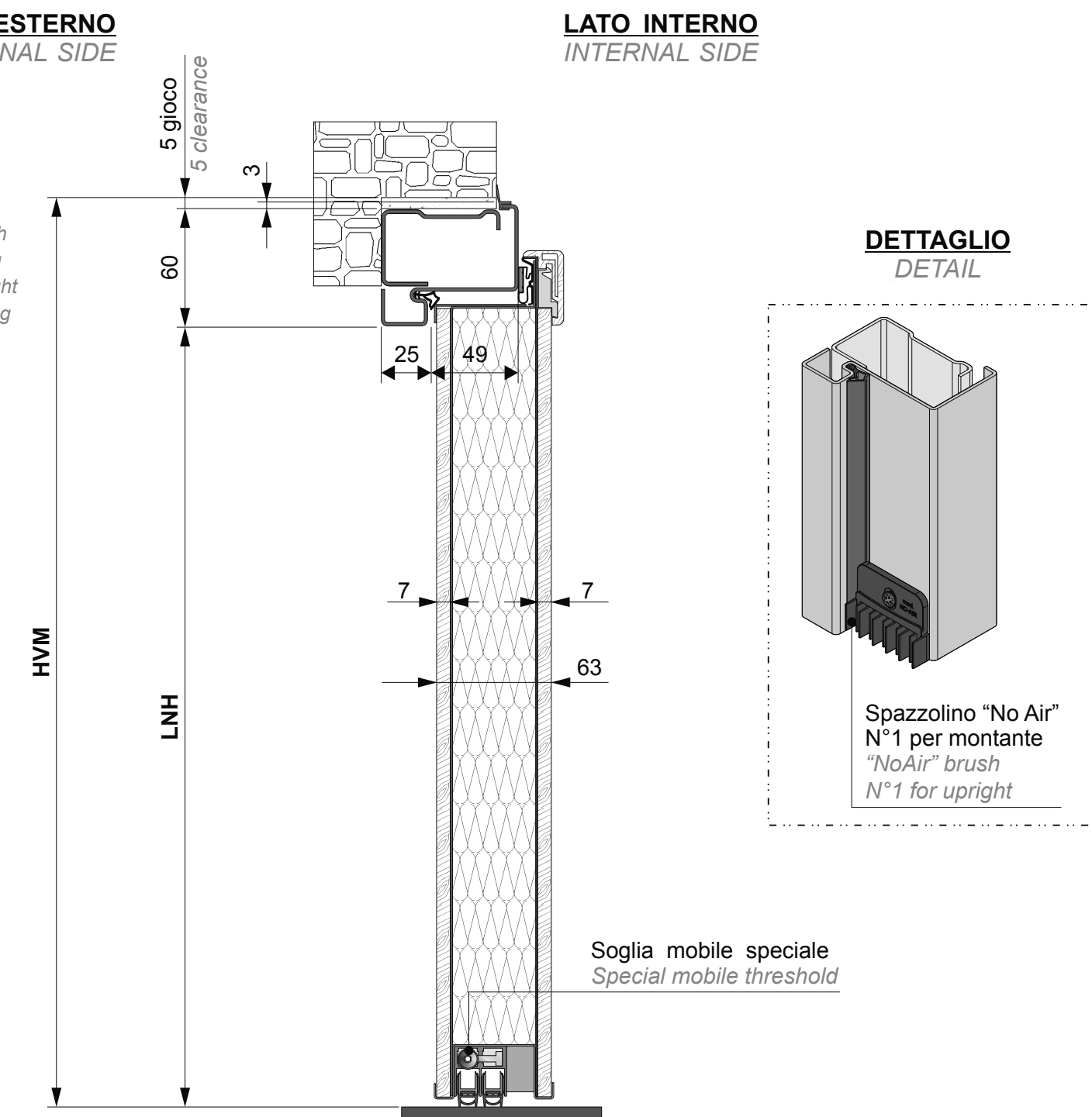
SEZIONE LONGITUDINALE - LONGITUDINAL SECTION
