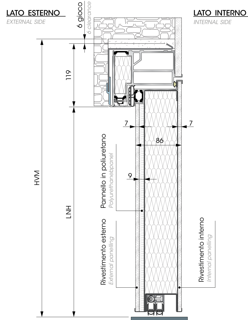
SEZIONE VERTICALE - VERTICAL SECTION
