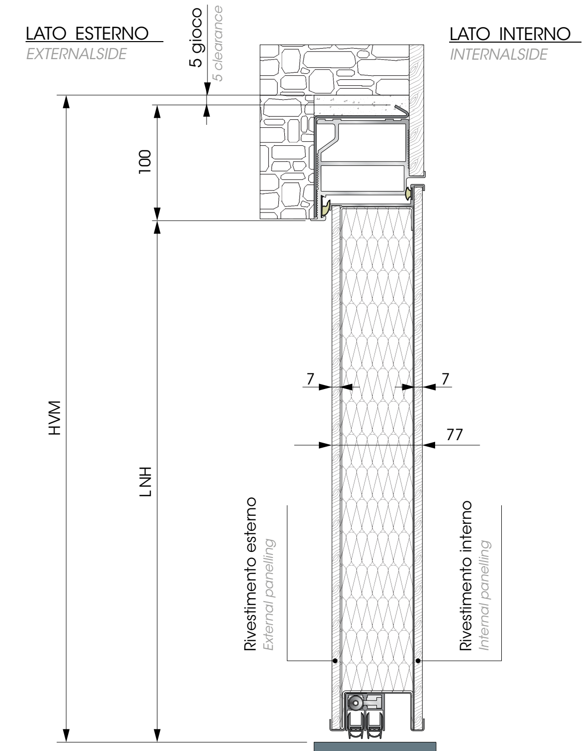
SEZIONE VERTICALE - VERTICAL SECTION
