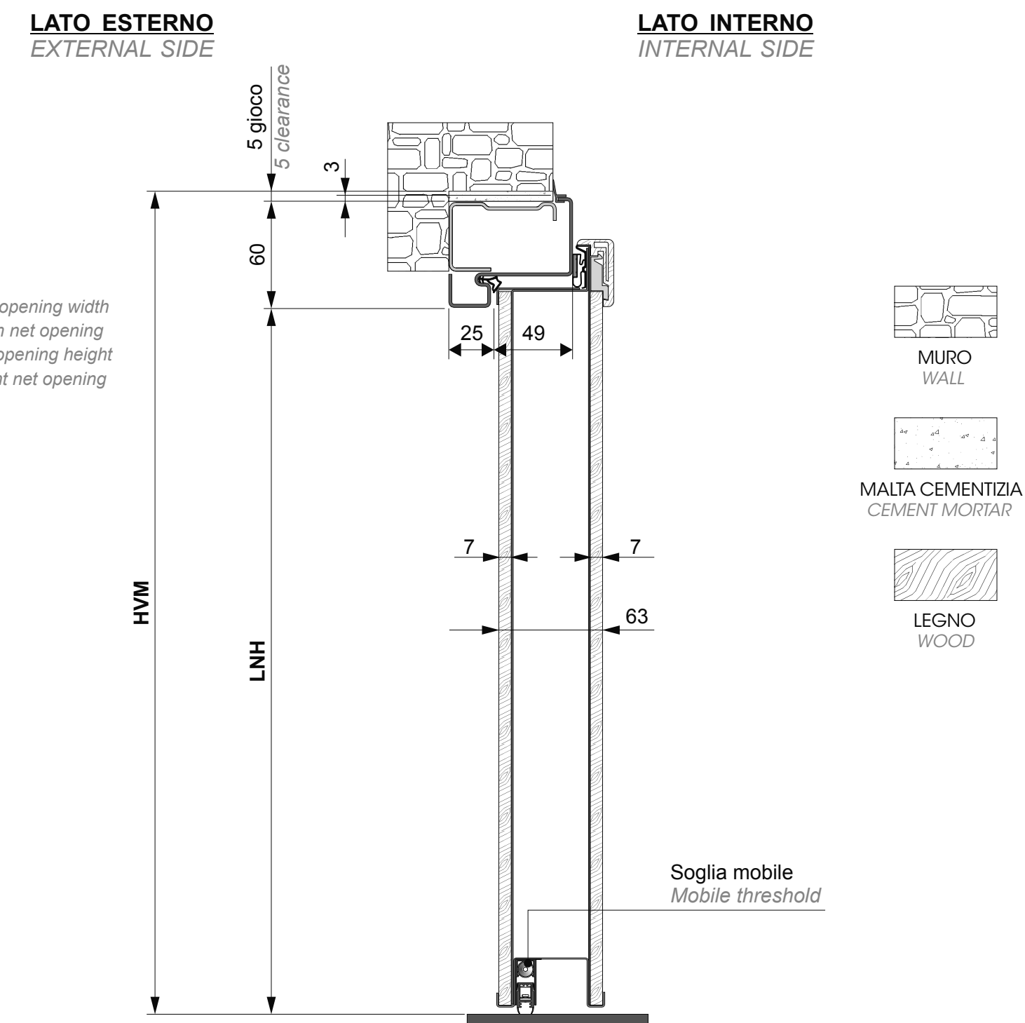
SEZIONE VERTICALE - VERTICAL SECTION
