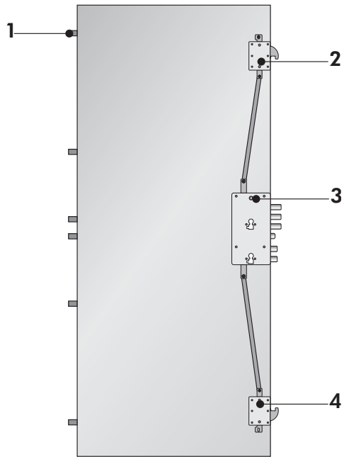
Synergy Out Sentry Doble
