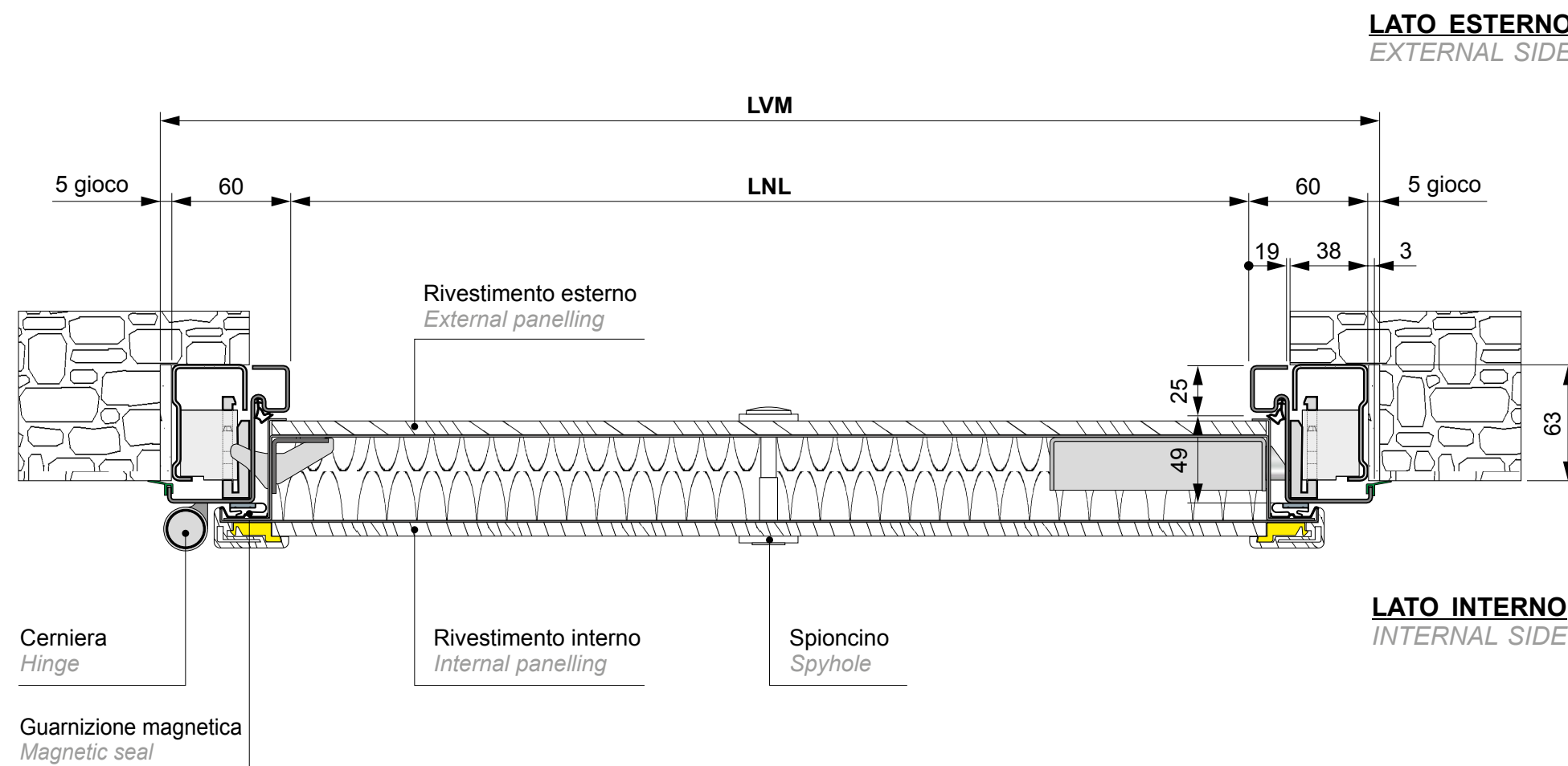
SEZIONE ORIZZONTALE - HORIZONTAL SECTION
