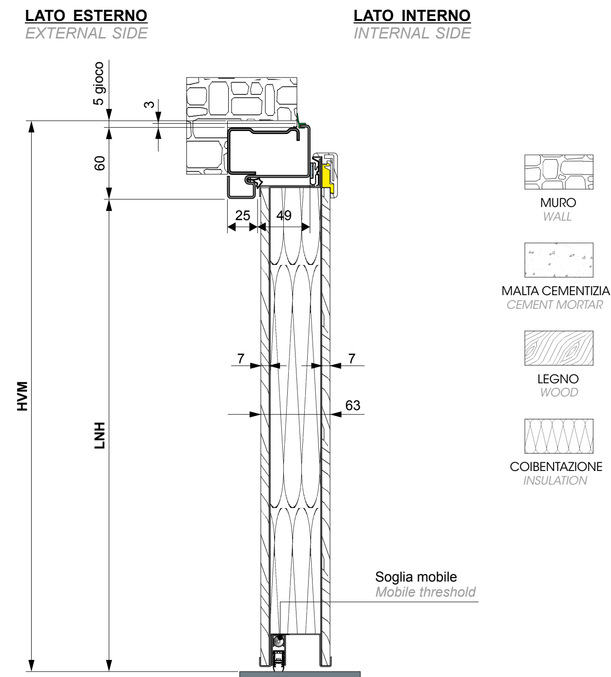
SEZIONE VERTICALE - VERTICAL SECTION
