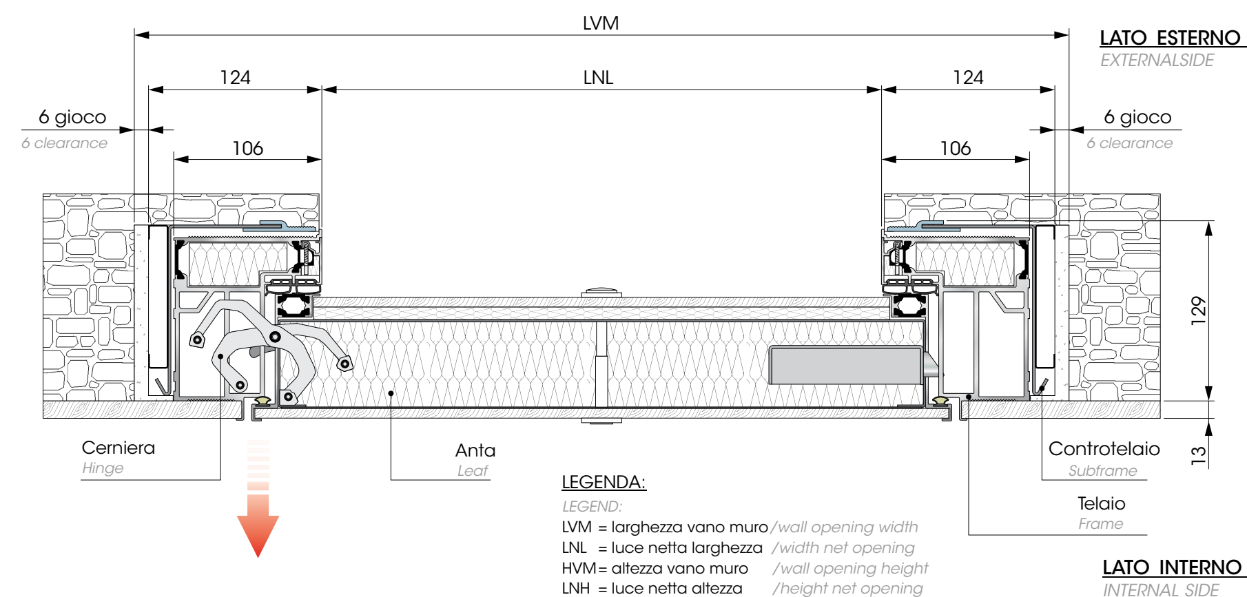
SEZIONE ORIZZONTALE - HORIZONTAL SECTION
