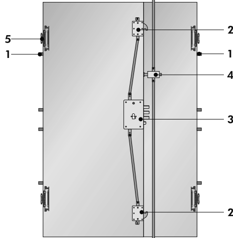
Sleek Sentry1 Doppio Battente - Double Leaf
