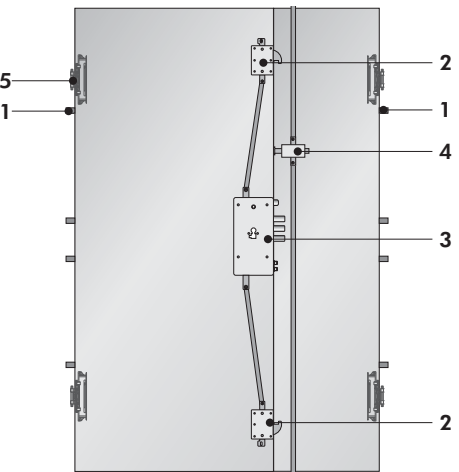
Sleek hibry5 Doppio battente - Double Leaf
