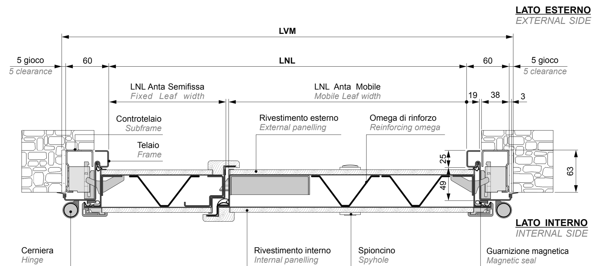
SEZIONE ORIZZONTALE - HORIZONTAL SECTION
