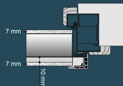
RIVESTIMENTI OPTIONAL - OPTIONAL PANELLING NEW TERMICO LINE E SUPER TERMICO LINE
