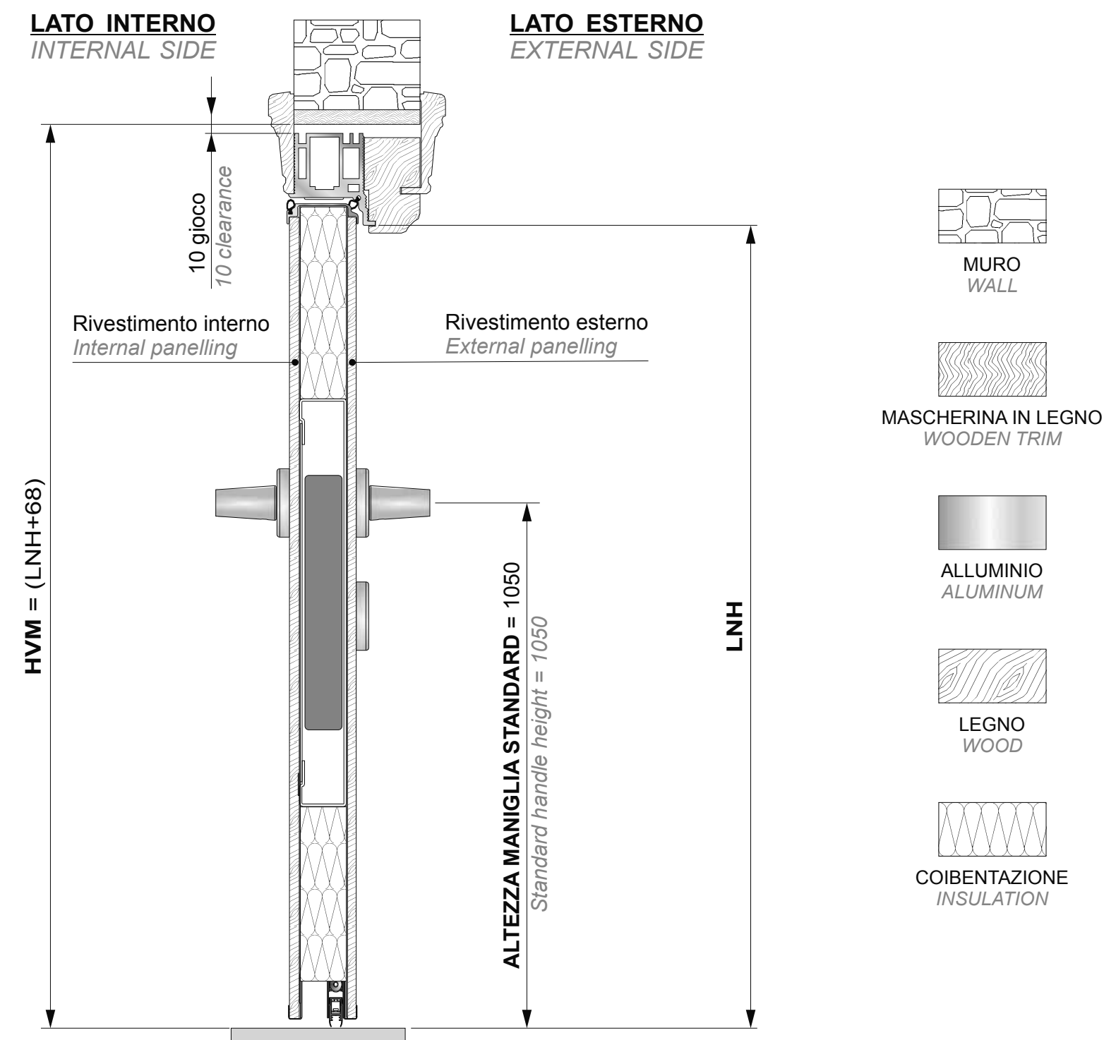
SEZIONE VERTICALE - VERTICAL SECTION
