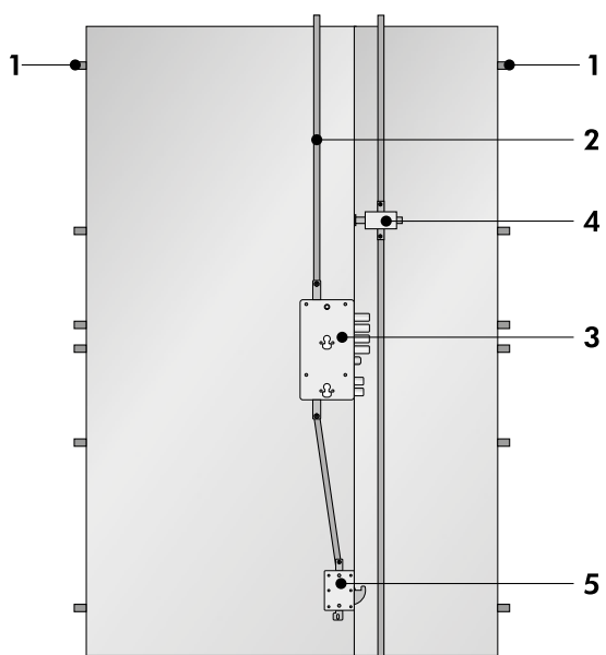
Sentry Doble D.B
