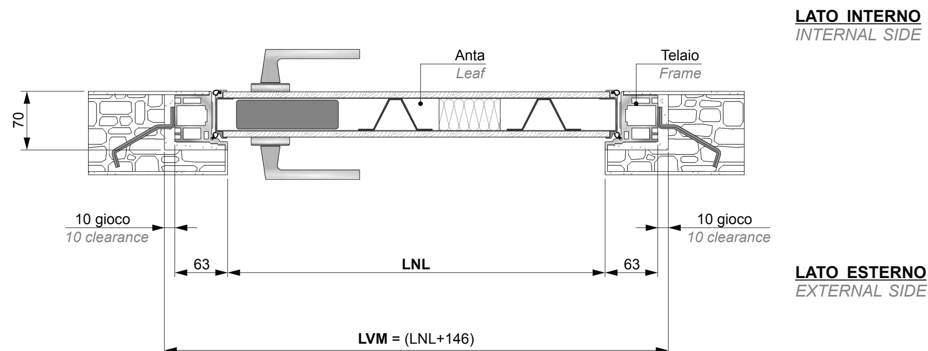
SEZIONE ORIZZONTALE - HORIZONTAL SECTION
