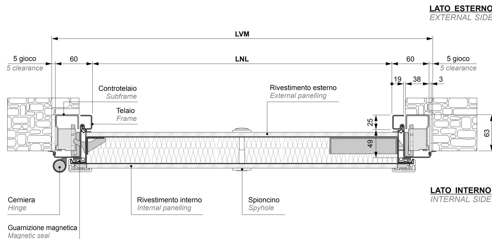
SEZIONE TRASVERSALE - CROSS SECTION
