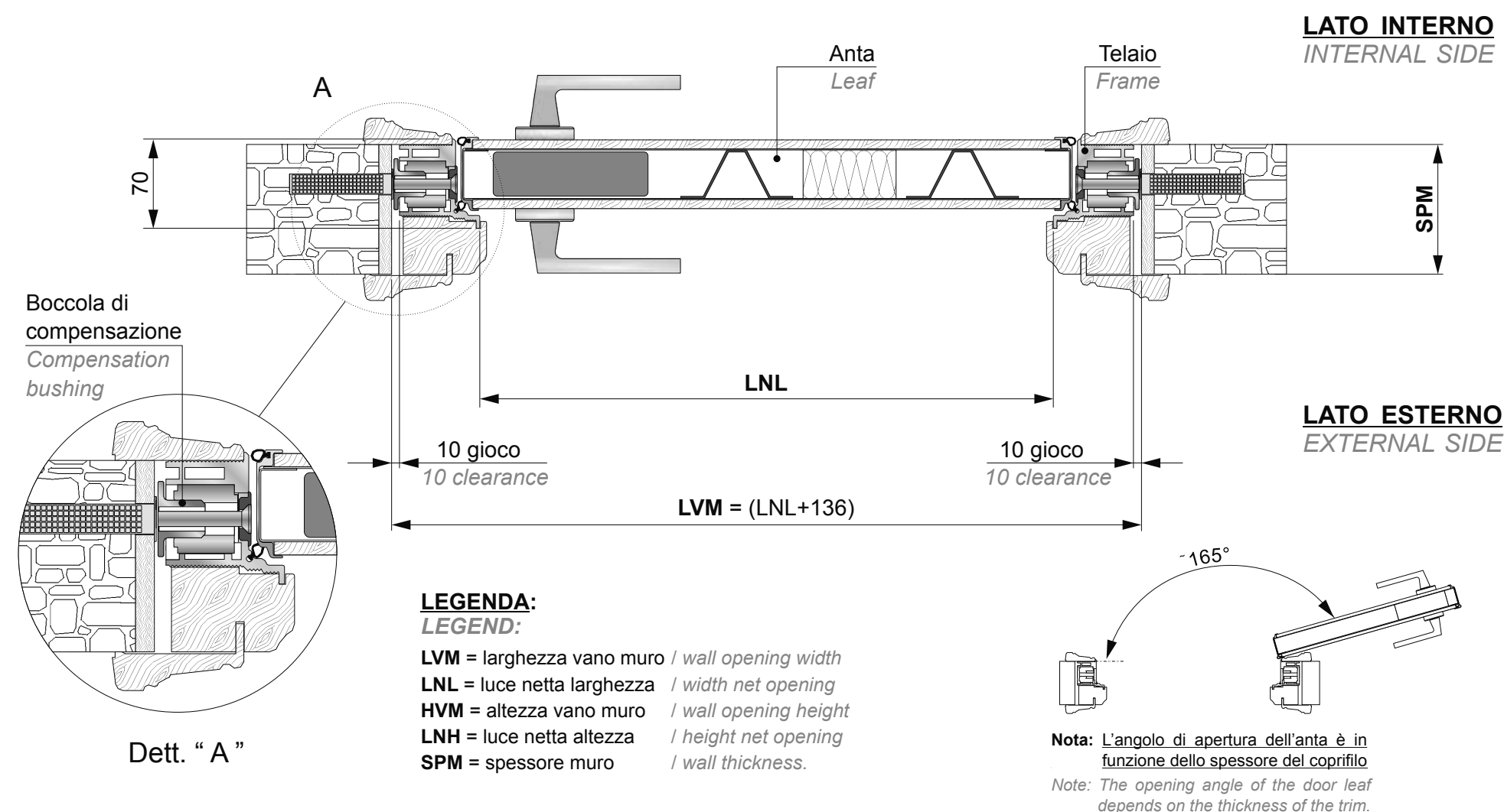
SEZIONE ORIZZONTALE - HORIZONTAL SECTION
