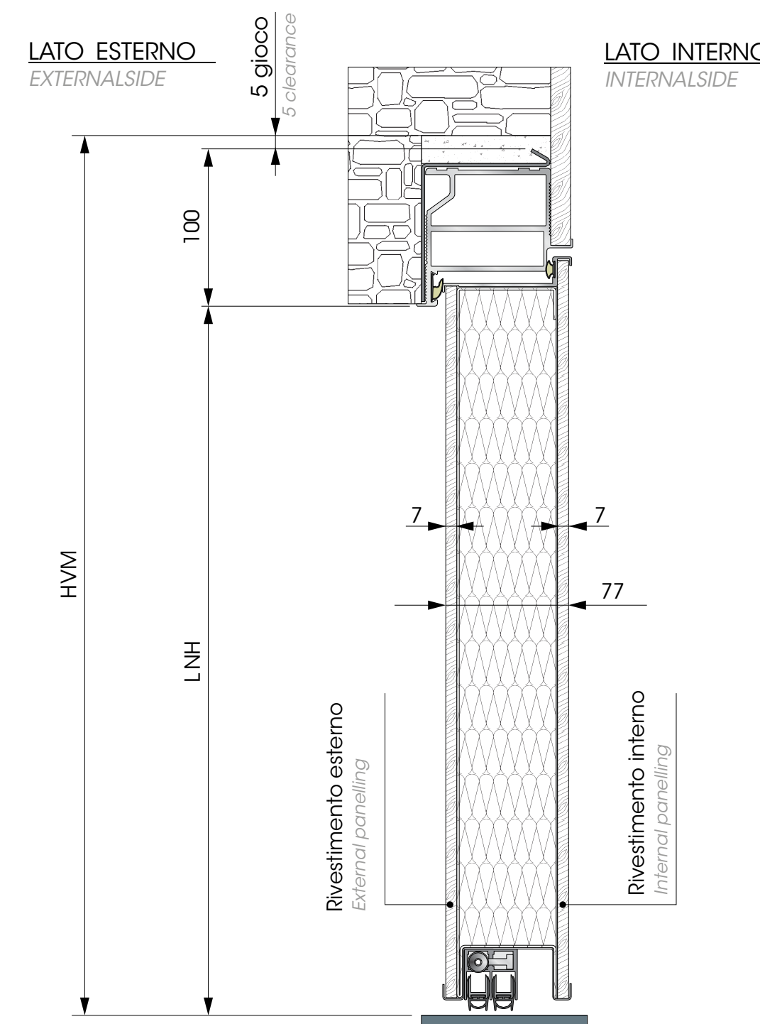
SEZIONE VERTICALE - VERTICAL SECTION
