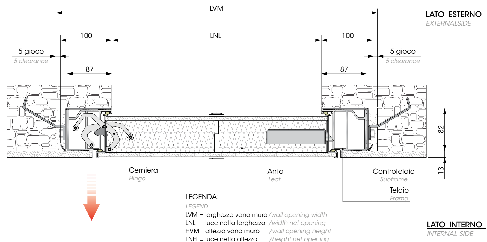
SEZIONE ORIZZONTALE - HORIZONTAL SECTION
