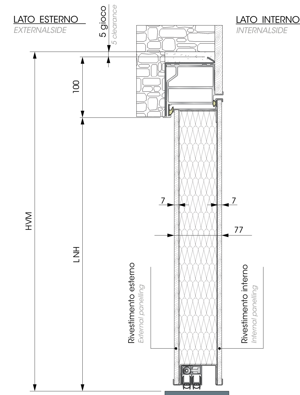
SEZIONE VERTICALE - VERTICAL SECTION
