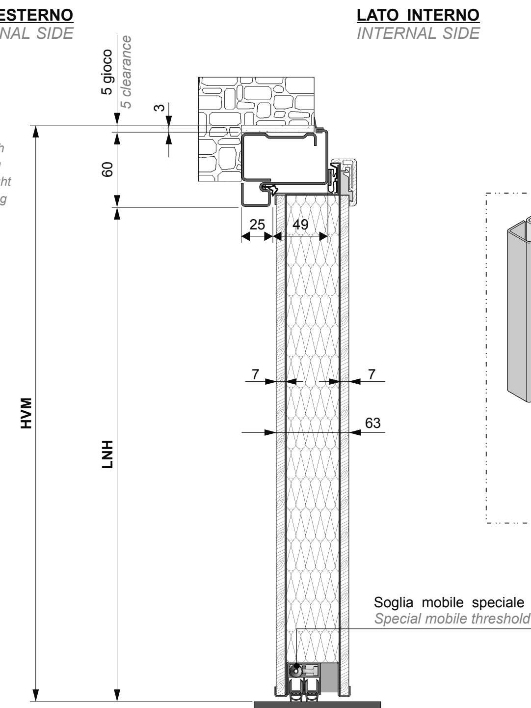
SEZIONE LONGITUDINALE - LONGITUDINAL SECTION
