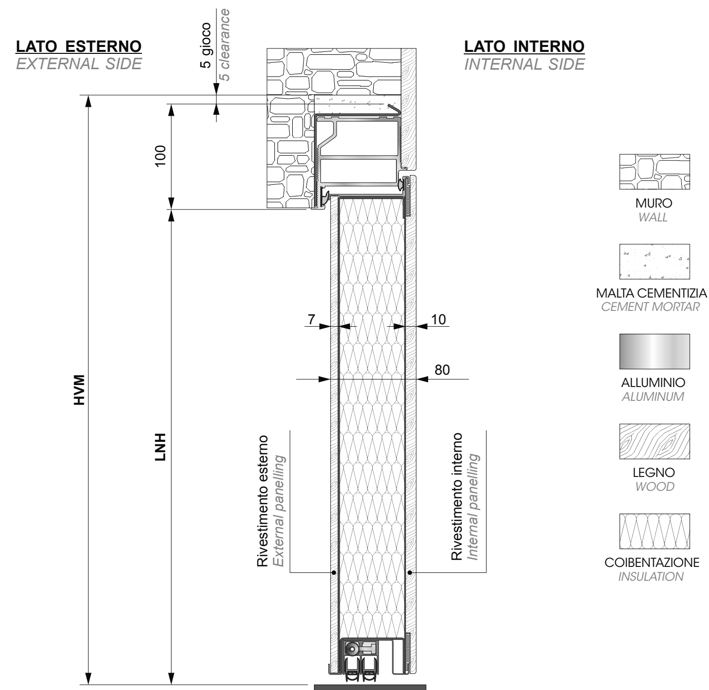
SEZIONE VERTICALE - VERTICAL SECTION
