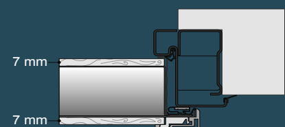
RIVESTIMENTI DI SERIE LISCI STANDARD FLUSH PANELLING
