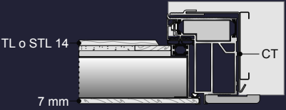
CT = Controtelaio TL = New termico line STL = Super termico line
