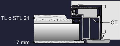
*Montati sul lato a spingere *Fitted on the push side
