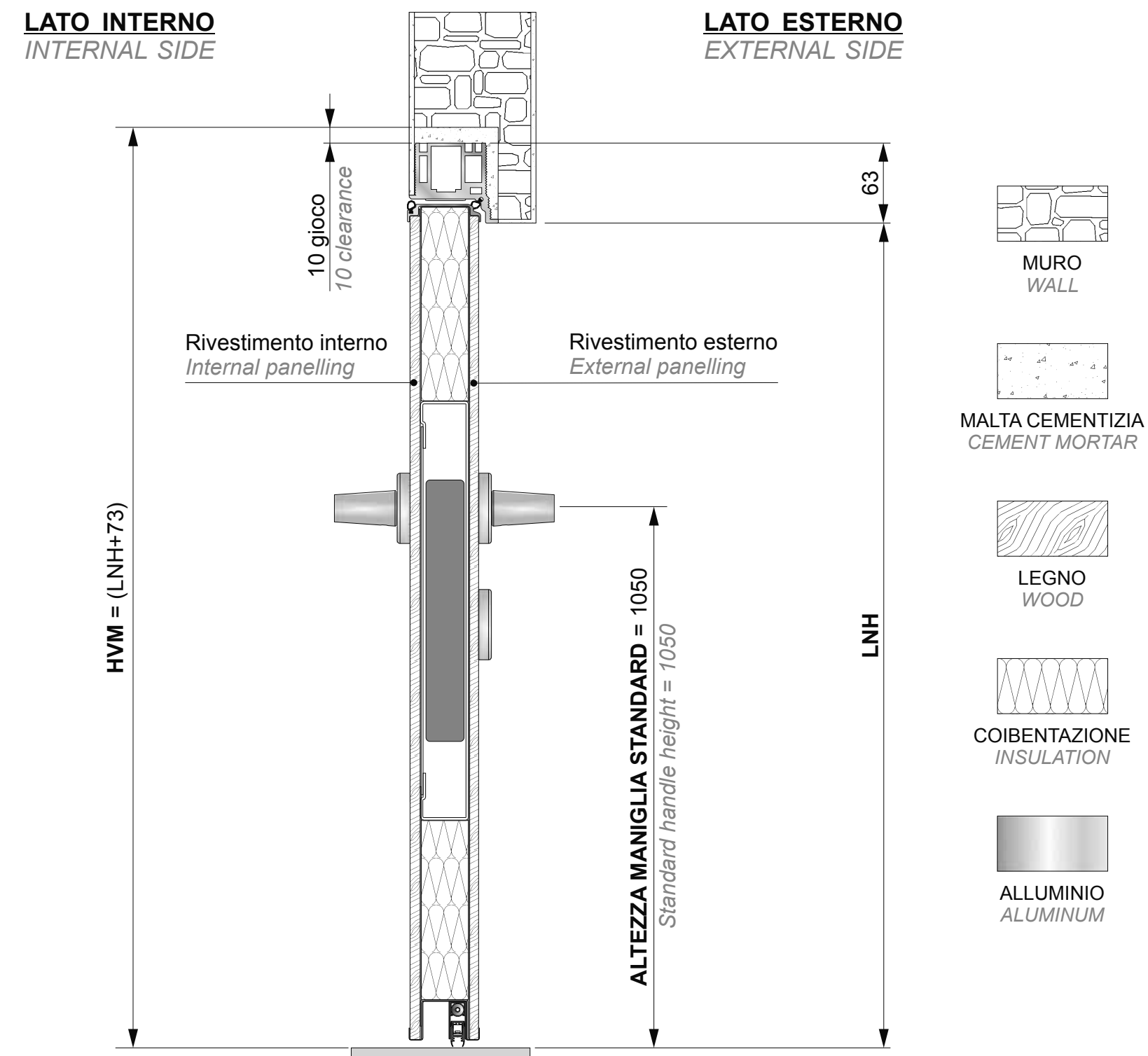
SEZIONE VERTICALE - VERTICAL SECTION
