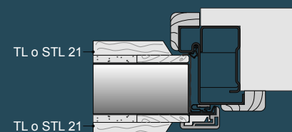
RIVESTIMENTI OPTIONAL - OPTIONAL PANELLING NEW TERMICO LINE E SUPER TERMICO LINE
