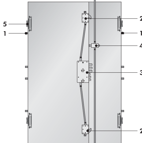
Sleek Sentry Doble Doppio Battente - Double Leaf
