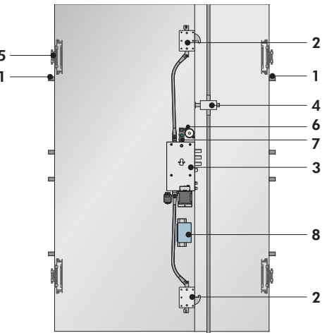
Sleek Next Elettra Doppio Battente - Double Leaf
