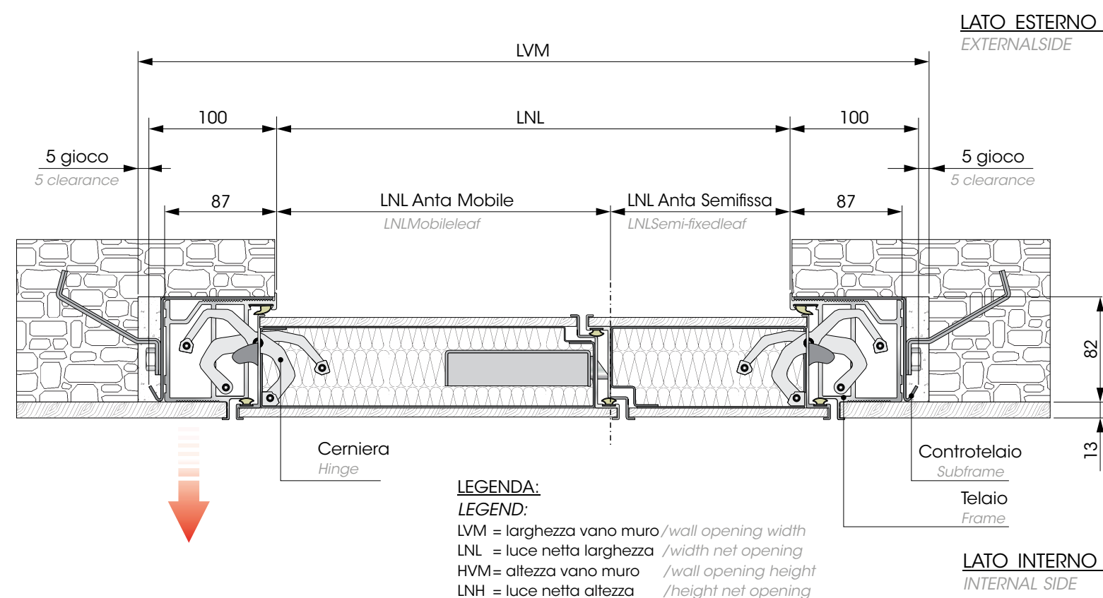
SEZIONE ORIZZONTALE - HORIZONTAL SECTION
