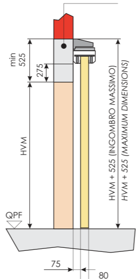
SENZA PORTINA PEDONALE WITHOUT PEDESTRIAN DOOR
