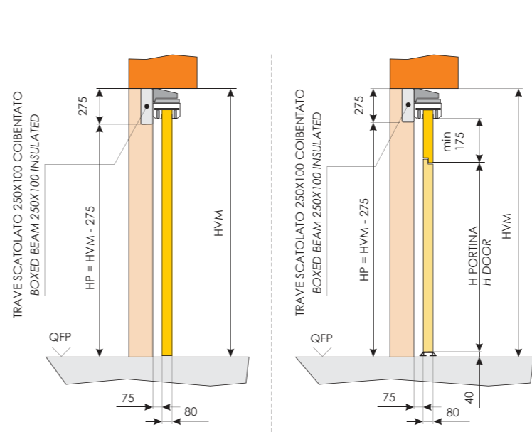
SENZA PORTINA PEDONALE WITHOUT PEDESTRIAN DOOR CON PORTINA PEDONALE WITH PEDESTRIAN DOOR
