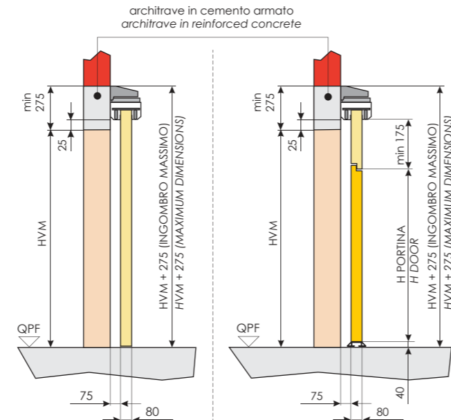
SENZA PORTINA PEDONALE WITHOUT PEDESTRIAN DOOR CON PORTINA PEDONALE WITH PEDESTRIAN DOOR
