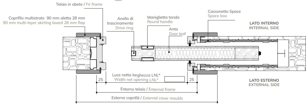
SEZIONE TRASVERSALE - CROSS SECTION
