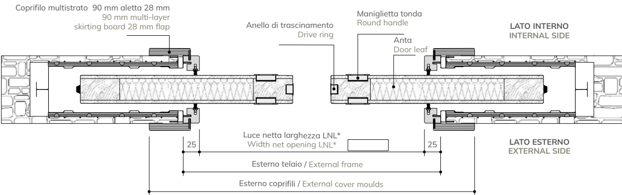
SEZIONE LONGITUDINALE - LONGITUDINAL SECTION
