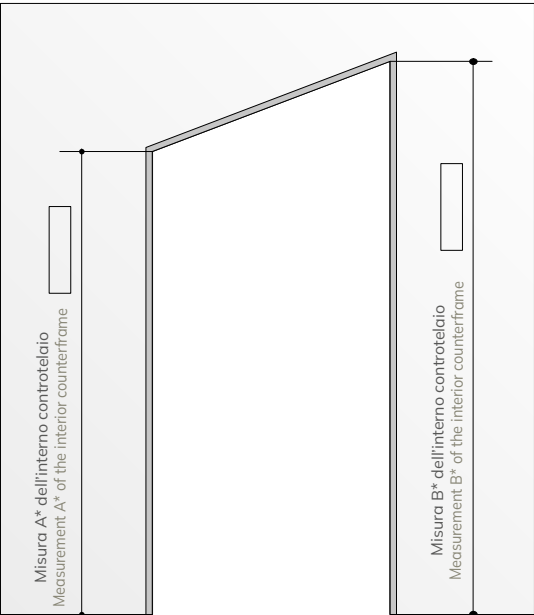
VISTA LATO ESTERNO - EXTERNAL VIEW
