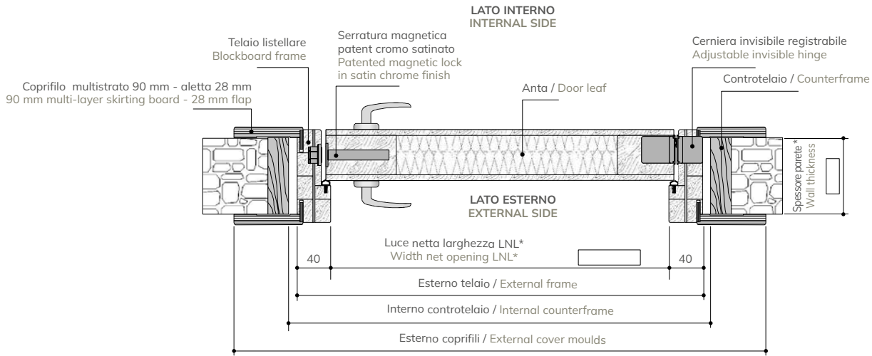
SEZIONE TRASVERSALE - CROSS SECTION
