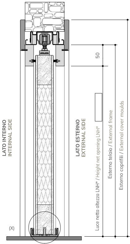
SEZIONE LONGITUDINALE - LONGITUDINAL SECTION
