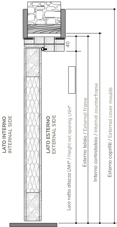
SEZIONE LONGITUDINALE - LONGITUDINAL SECTION
