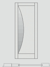
Sezione orizzontale anta Leaf horizontal section
