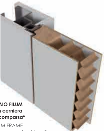
TELAIO FILUM REVERSE con cerniera a scomparsa reversibile* FILUM REVERSE FRAME with concealed reversible hinge*
